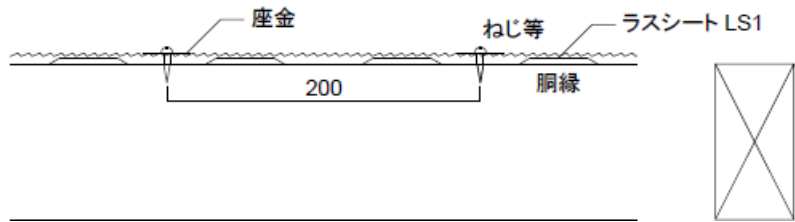
図 14 木造でのラスシート LS1 の留め付け
