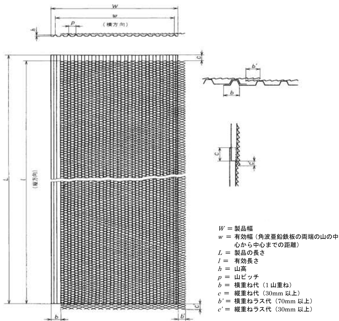
図 1 ラスシートの形状と呼び名
